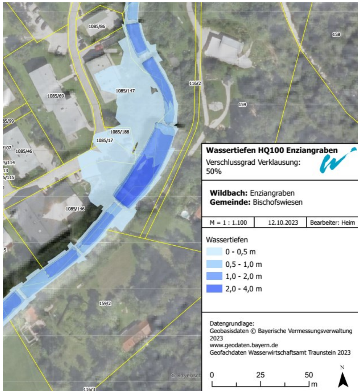
Abb. 5 Untersuchung Wassertiefen Enziangraben, Planungszustand Hochwasserschutz mit Ableitung des Wassers aus dem Maiswandgraben in den Enziangraben Quelle: WWA Traunstein
