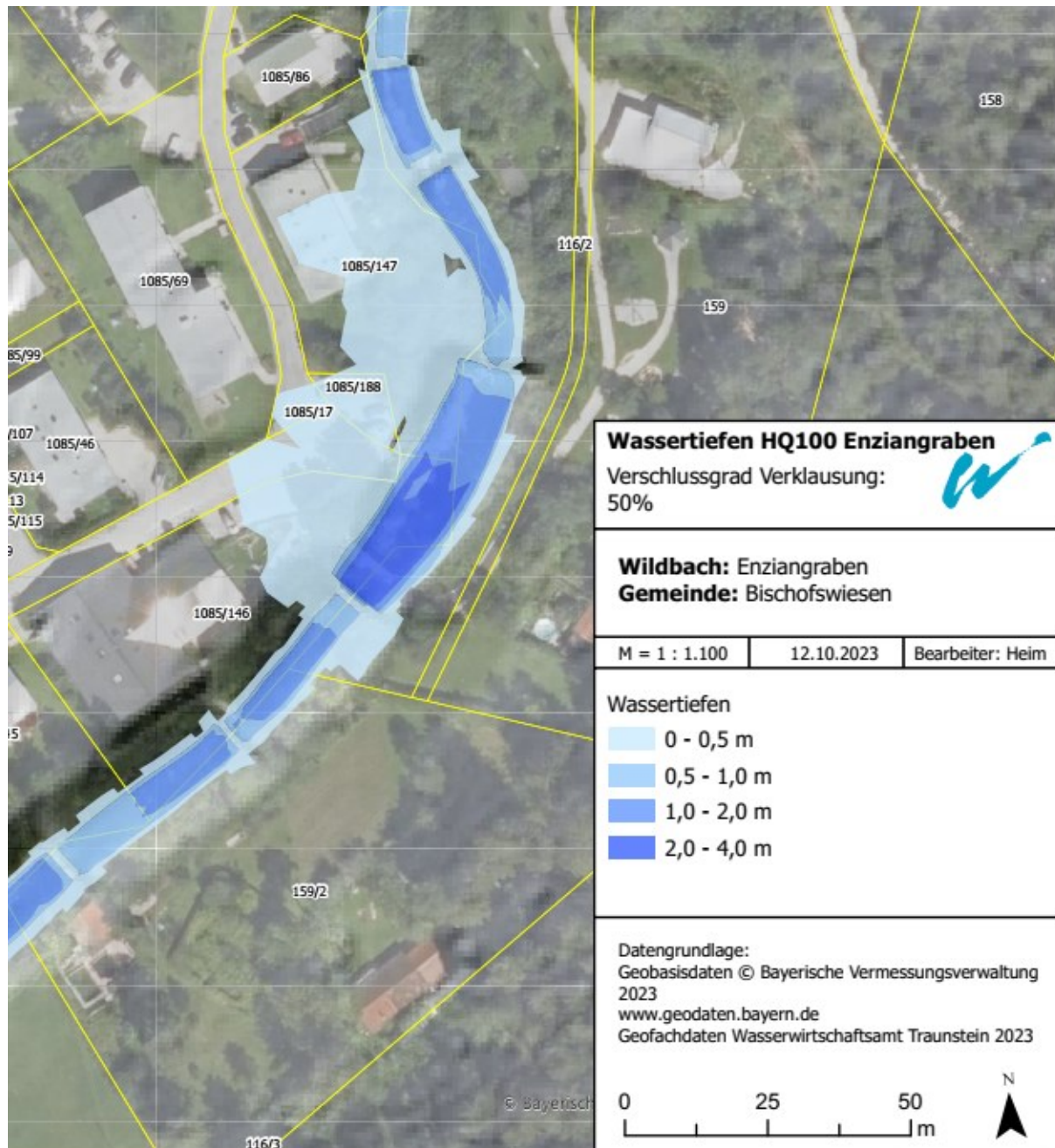
Abb. 9 Untersuchung Wassertiefen Enziangraben, Planungszustand Hochwasserschutz mit Ableitung des Wassers aus dem Maiswandgraben in den Enziangraben Quelle: WWA Traunstein
